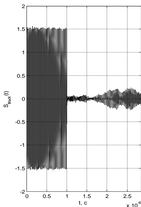
Рис.4. Отраженный от поверхности радиосигнал
