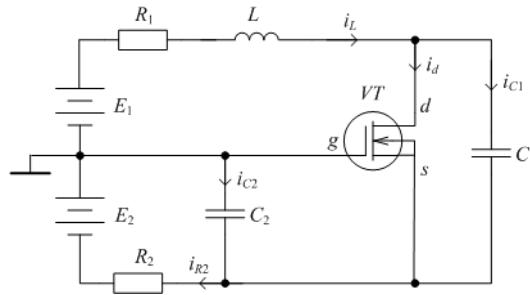
Рис. 1. Генератор хаотических колебаний на полевом транзисторе
