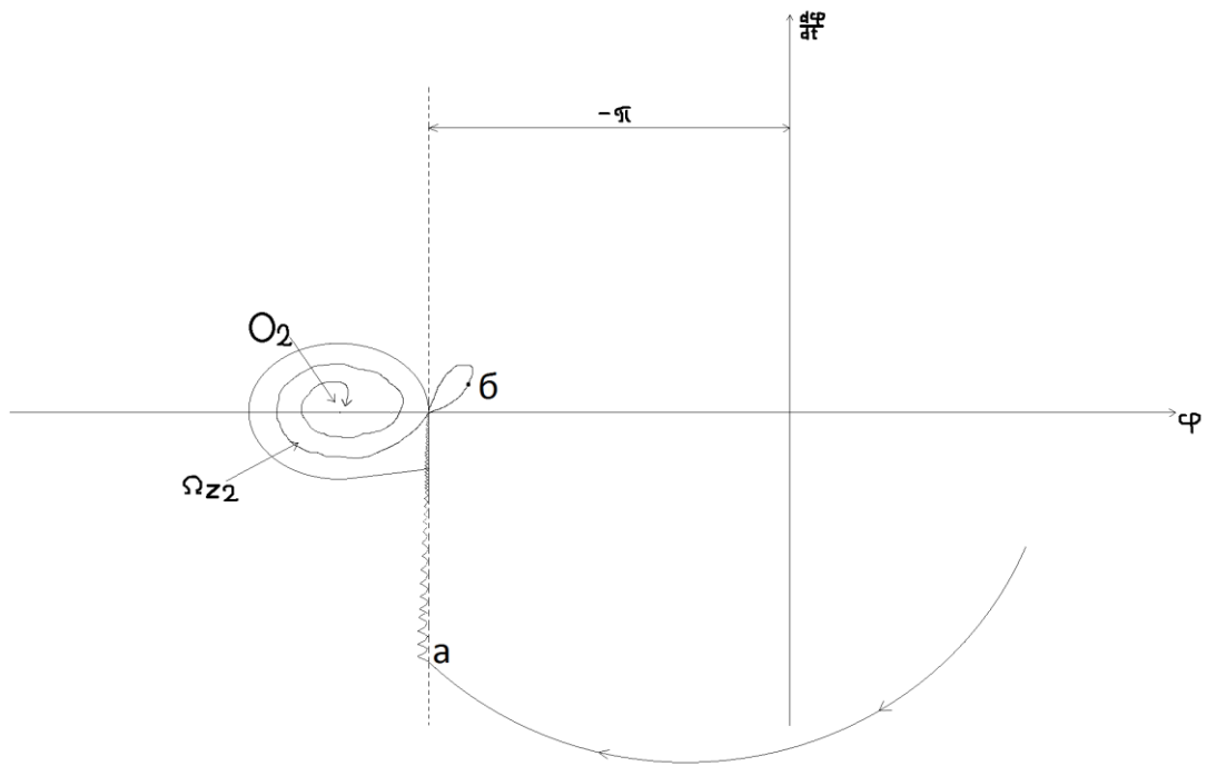
Рис.2. Фазовый портрет в системе ФАПЧ с дуальным управлением процессами.
