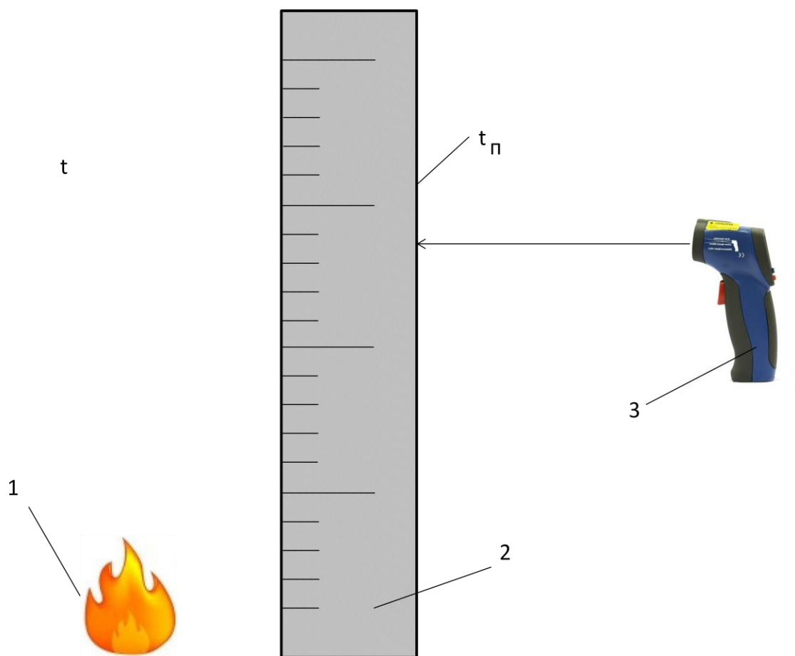
Рис.2. Методика проведения замеров: 1 – очаг пожара; 2- пробник «алюминиевая пластина»; 3 –лазерный пирометр
