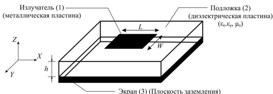
Рис.1. Модель микрополосковой антенны
