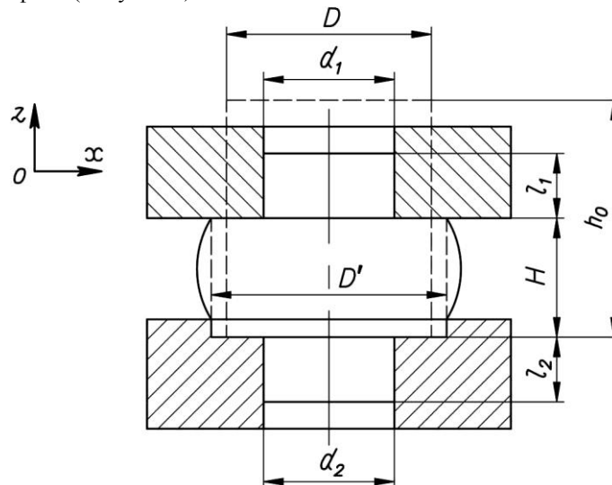
Рис.1. Схема двустороннего прессования в открытом штампе
