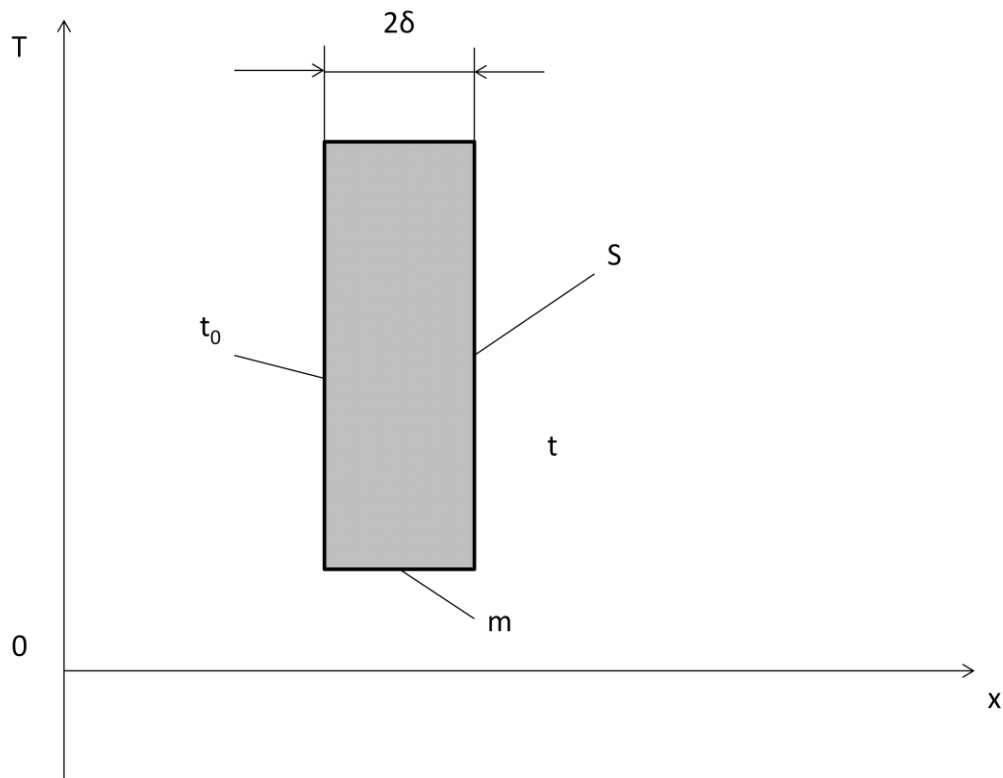
Рис.3. Теплопередача через плоскую стенку
