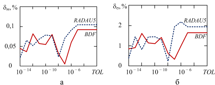
Рис.4. Зависимости модулей относительных погрешностей оценки математического ожидания (а) и СКО (б) выходного напряжения от значения TOL
