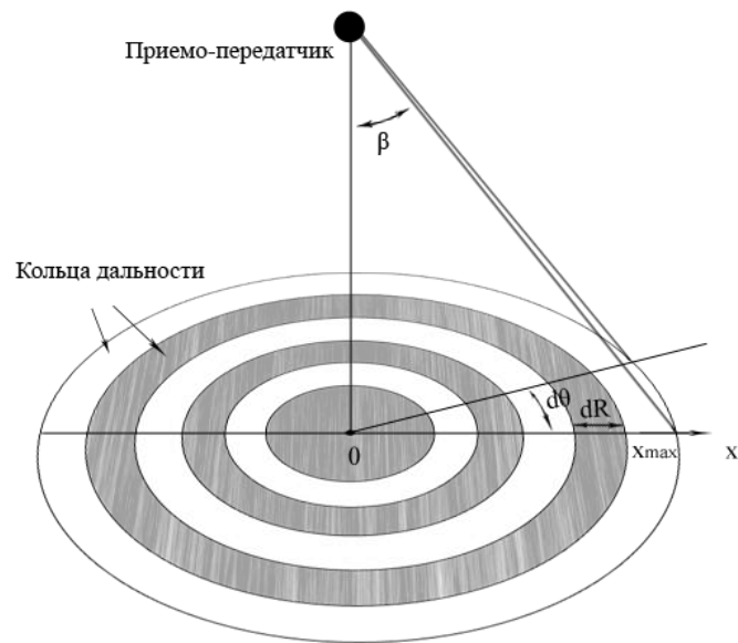
Рис.2. Формирование колец дальностей на подстилающей поверхности
