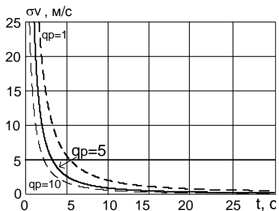
Рис.3. Зависимость СКО координаты Ула от времени наблюдения
