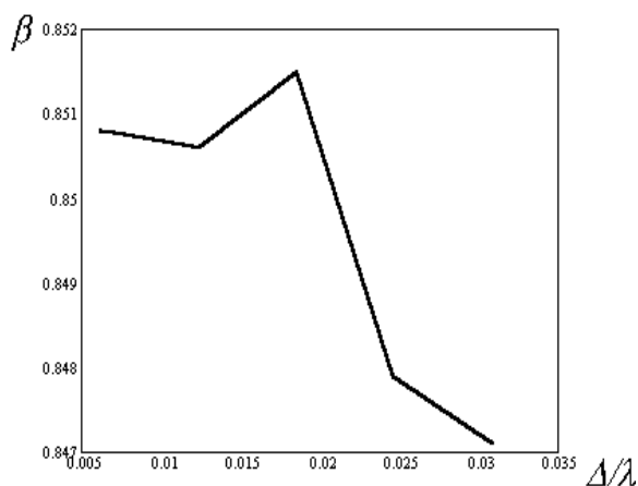
Рис.3. Зависимость \beta при равномерном законе распределения ошибки изготовления профиля рефлектора
