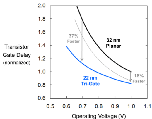
Рис.4. Быстродействие планарных и Tri-Gate транзисторов
