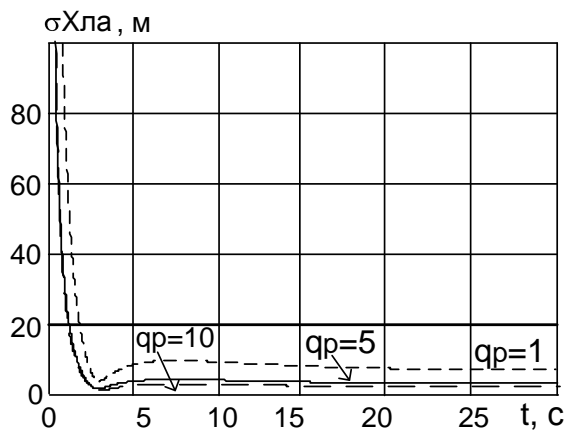
Рис.2. Зависимость СКО координаты Хла от времени наблюдения
