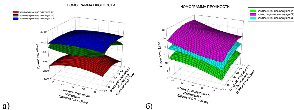
Рис.1. Зависимость плотности (а) и прочности (б) раствора от содержания: композиционного вяжущего, наполнителя (отхода флотационного обогащения железных руд фракции 0...0,315мм) и мелкого заполнителя (отхода флотационного обогащения железных руд фракции 0,5...0,9 мм)
