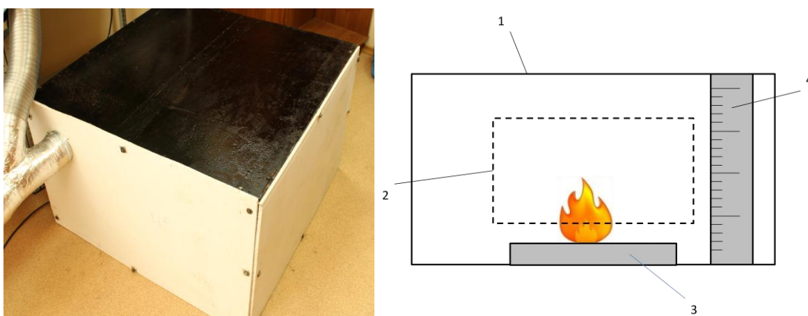
Рис.1. Фотография и схема модельной экспериментальной установки: 1 – камера сгорания; 2 – проем; 3 – очаг пожара; 4 – алюминиевая пластина.
