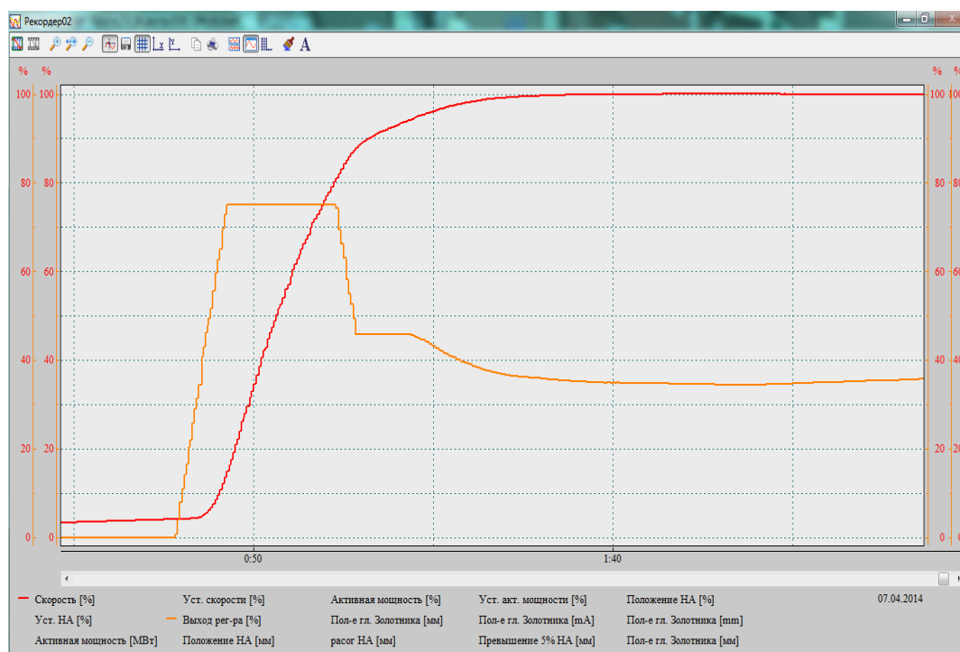
Рис.1. Экспериментальная переходная характеристика разгона гидрогенератора.
