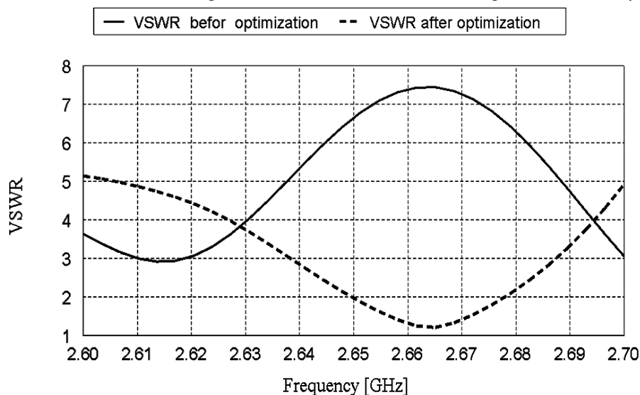
Рис.4. Частотная зависимость КСВ для микрополосковой антенной решетки до и после оптимизации
