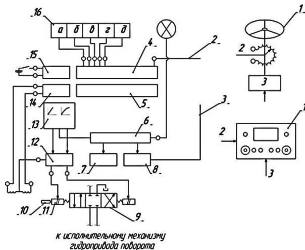
Рис.4. Блоксхема системы электронно – гидравлического управления поворотом:
