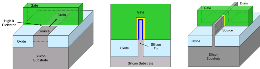
Рис.2. Схемы трехмерной структуры транзисторов
