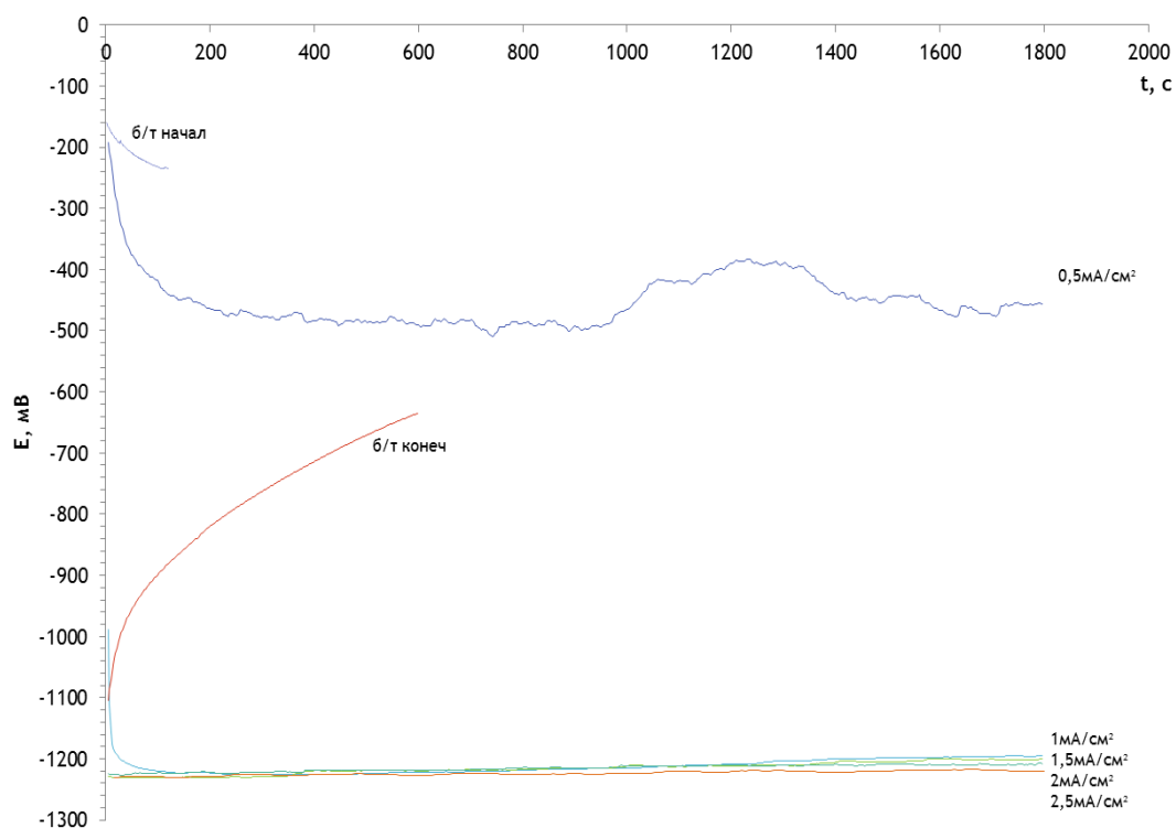
Рис.3. Влияние плотности тока на ход катодных гальваностатических кривых медного электрода в 0,1моль/л растворе \text{Na}_2\text{MoO}_4 .
