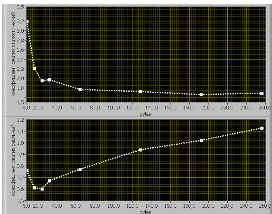
Рис.2. Зависимость коэффициентов сжатия от количества байт кодируемой информации
