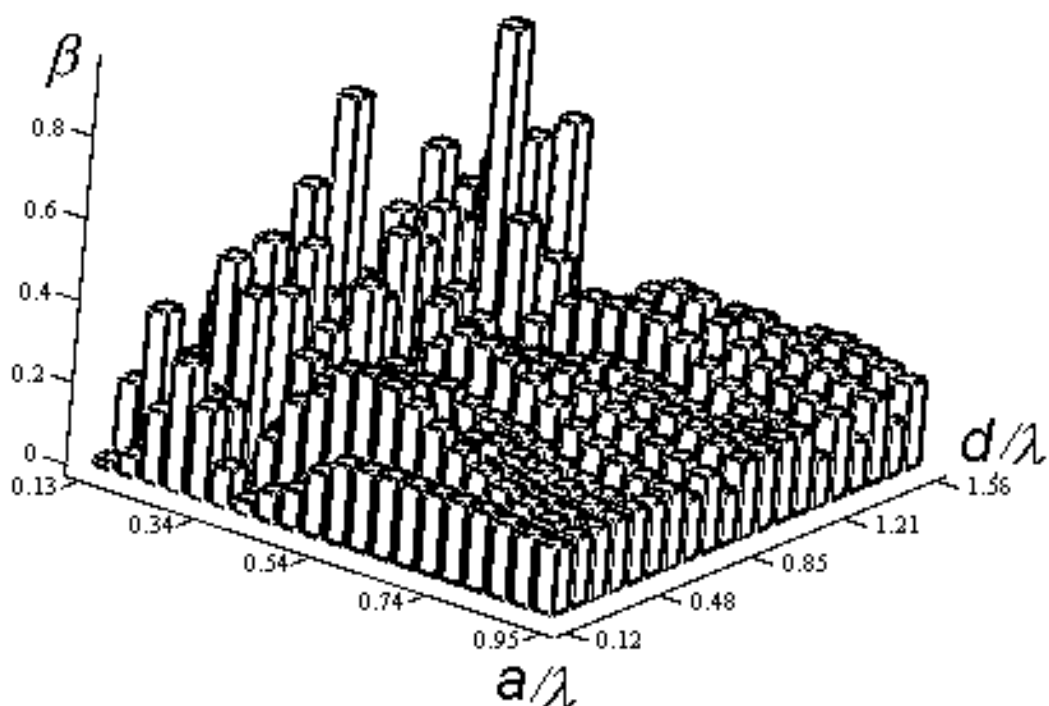
Рис.1. Зависимость коэффициента равномерности КАР от параметров компоновки
