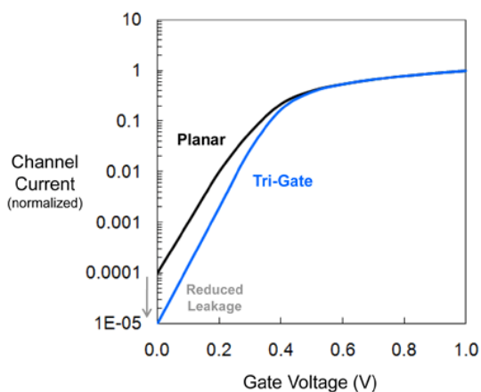
Рис.3. Сравнение зависимости тока утечки от напряжения у Tri-Gate и планарного транзисторов
