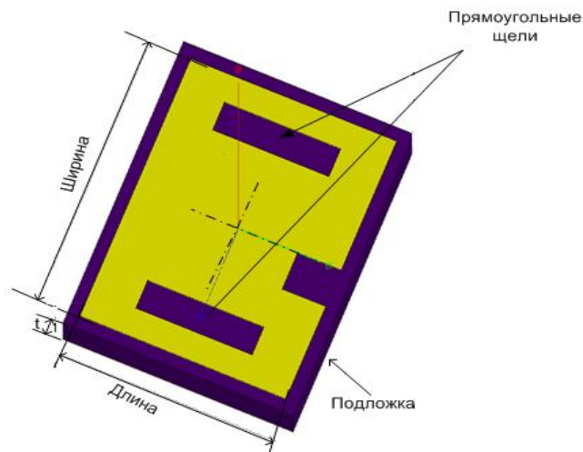
Рис.2. Геометрия одного элемента излучателя МПАР
