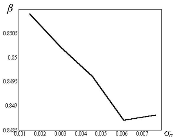
Рис.4. Зависимость \beta при нормальном законе распределения ошибки изготовления профиля рефлектора
