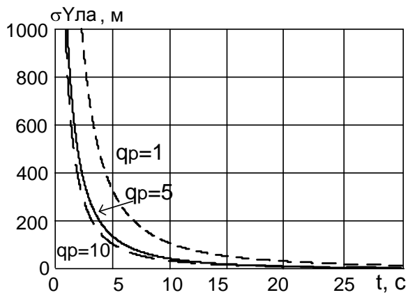
Рис.3. Зависимость СКО координаты Ула от времени наблюдения
