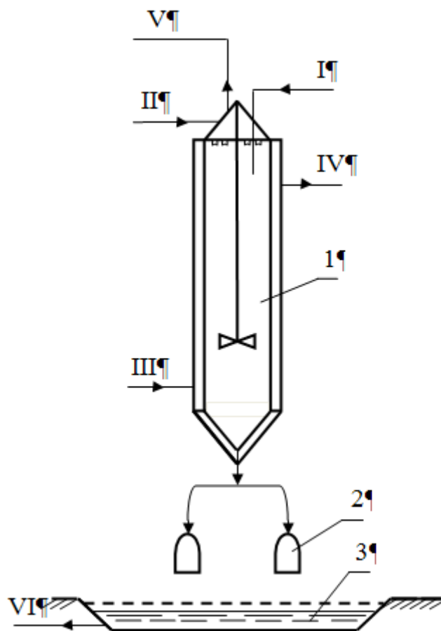
Рис.1. Принципиальная схема блока гранулирования
