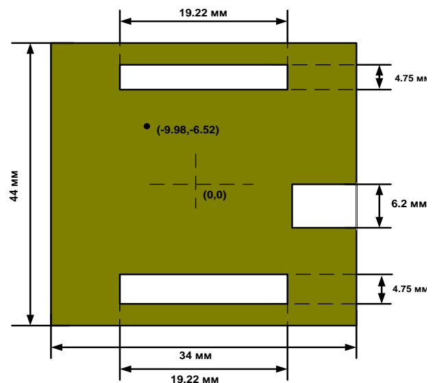
Рис.3. Проект одного элемента излучателя МПАР
