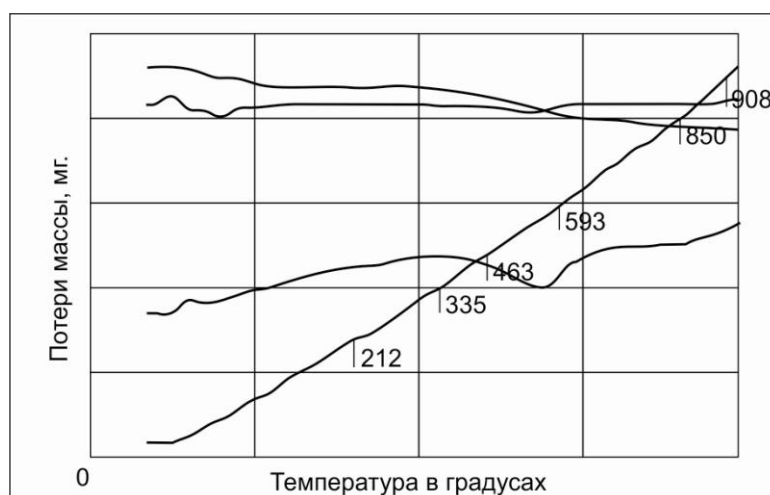
Рис.1. Термограммы алевролитовых пород
