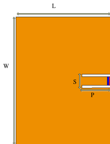
Рис.1. Конфигурация микрополосковой антенны
