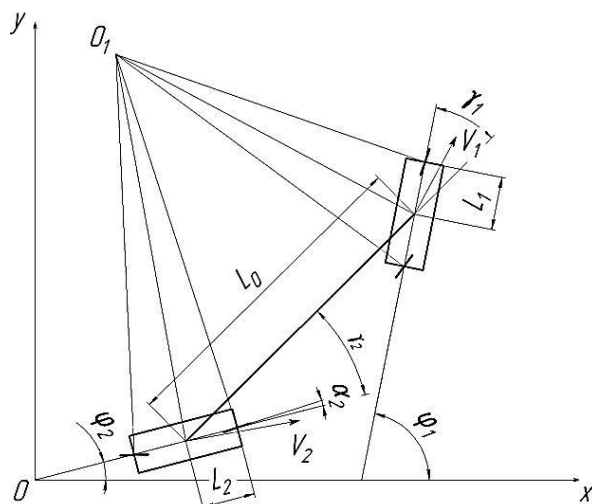
Рис.5. Схема движения автопоезда на платформах, работающих на некотором расстоянии друг от друга.
