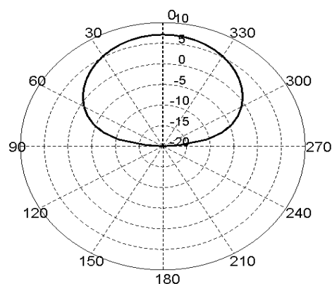
Рис.3. Коэффициент усиления антенны на частоте 2.4ГГц
