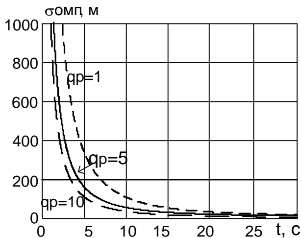
Рис.6. Зависимость СКО местоположения от времени наблюдения
