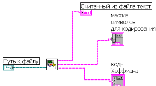
Рис.1. Библиотечный модуль – вложенный виртуальный прибор кодера Хаффмана
